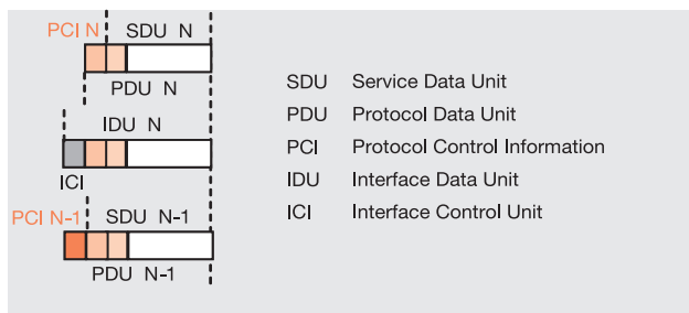
Bild 1.7 Schnittstellen und Dateneinheiten im OSI-Modell
