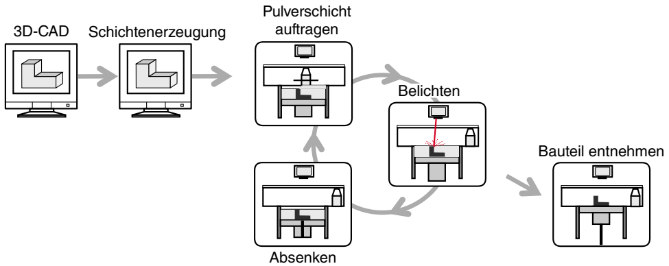
Bild 1.1 Prinzip der Additiven Fertigung am Beispiel eines pulverbettbasierten Laserverfahrens [Quelle: ETHZ pd/z, nach Poprawe 2005]
