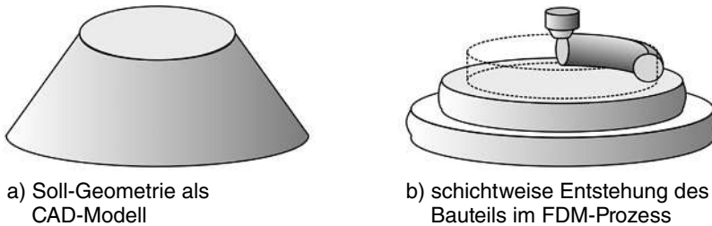
Bild 1.5 Schichtweiser Aufbau eines Bauteils im FDM-Prozess [Quelle: ETHZ pd|z]
