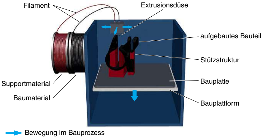
Bild 1.4 Aufbau einer FDM-Anlage [Quelle: ETHZ pd|z]
