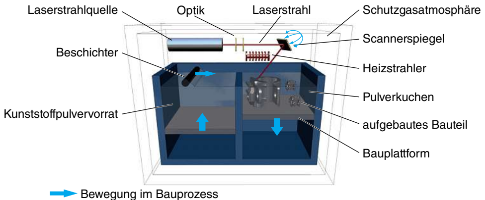
Bild 1.7 Aufbau einer Anlage zum Lasersintern [Quelle: ETHZ pd|z]
