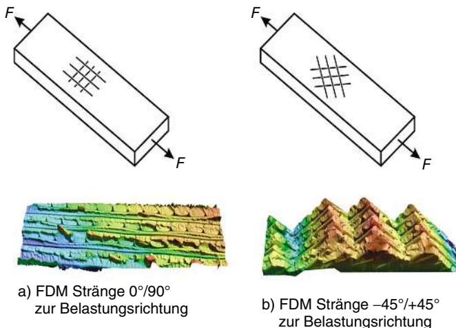
Bild 1.6 Bruchflächen von FDM-Zugproben bei unterschiedlichen Belastungsrichtungen relativ zur Strangrichtung [Quelle: ETHZ pd/z]
