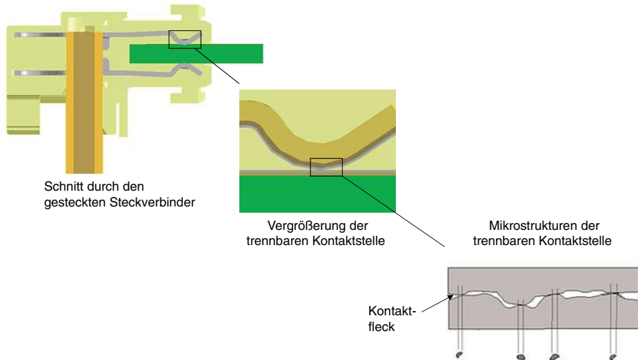
Bild 6.1 Analyse eines Kontaktpunktes
