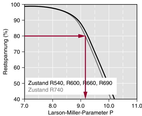
Bild 5.2 Bei einem Grenzwert von 80% erhält man z.B. für Bronze CuSn8 einen Larsson-Miller Parameter von 9,1.
