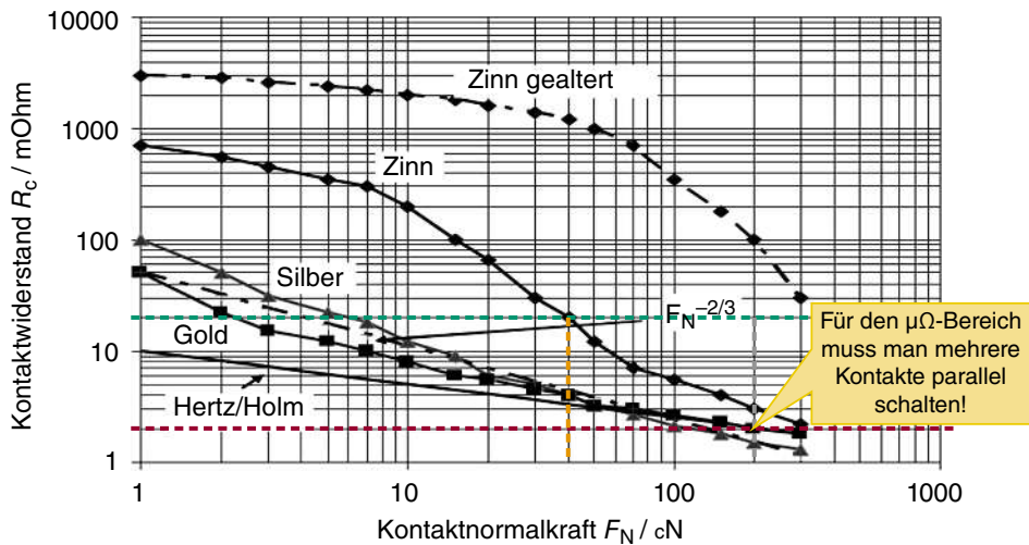
Bild 8.2 Kontaktwiderstand in Abhängigkeit der Kontaktnormalkraft für unterschiedliche Oberflächen [Q.4]
