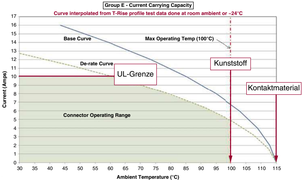
Bild 8.4 Ermittlung einer Deratingkurve nach IEC / EN 60 512-5-2
