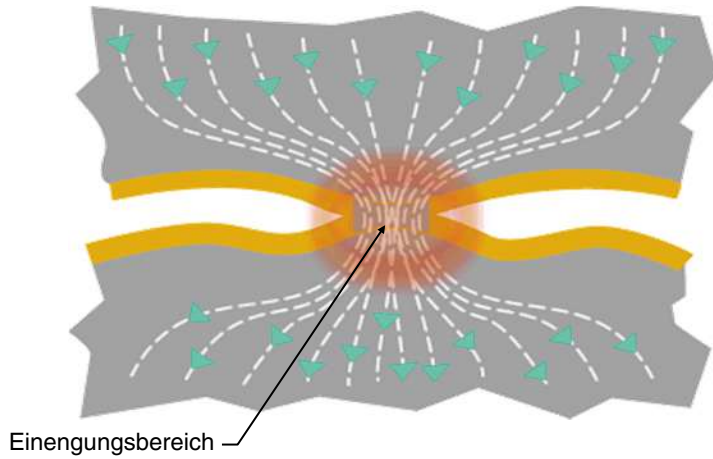
Bild 6.3 Strombündelung im Einengungsbereich
