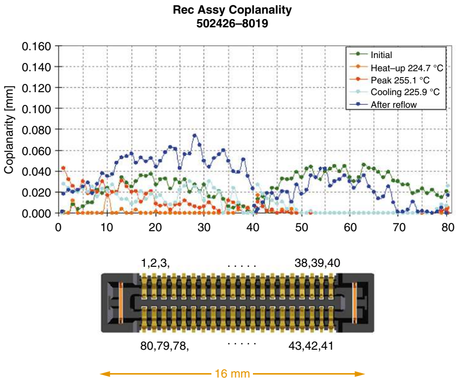
Bild 4.4 Krematoriumseffekt von Steckverbindern mit LCP-Gehäuse während des Reflow-Prozesses
