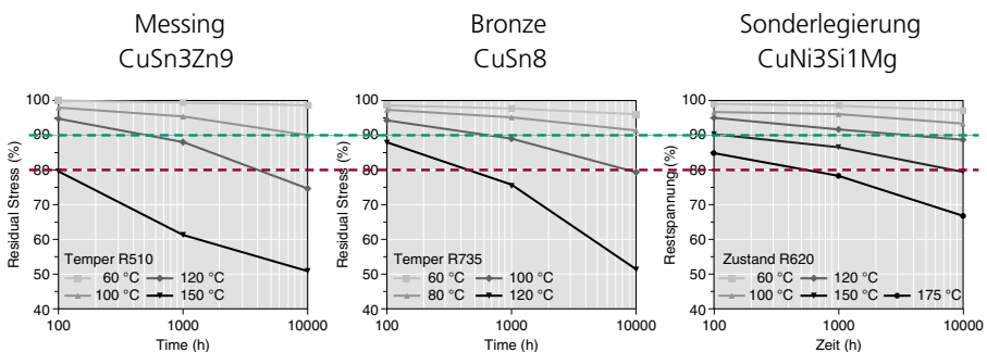
Bild 5.1 Unterschiedliche Relaxation bei Messing, Bronze und Sonderlegierung [Q.2]
