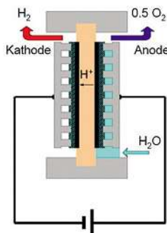
Bild 7.3 Funktionsprinzip PEM-Elektrolyse
