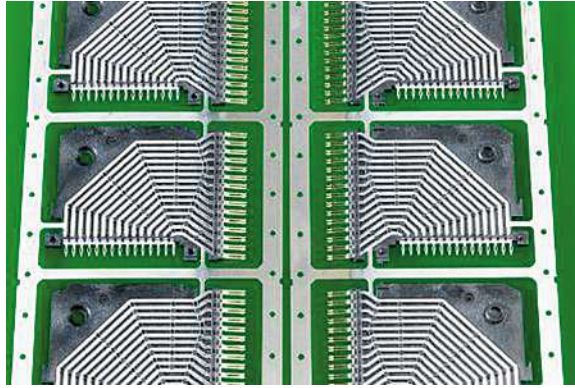
Bild 4.3 Diese Technik erlaubt es, u.a. ein Dielektrikum aus Luft zwischen einem differentiellen Paar aufzubauen, das exzellente Hochfrequenzeigenschaften hat.
