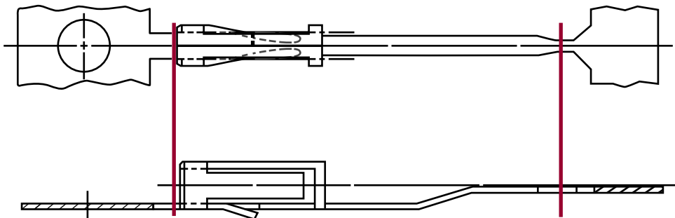
Bild 7.1 Offene Stanzkanten im Kontakt- und Einlötbereich
