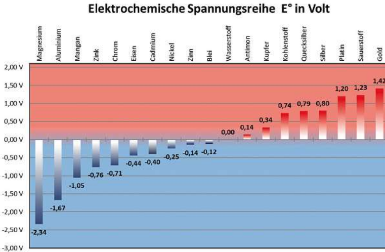
Bild 7.2 Elektrochemische Spannungsreihe E° in Volt
