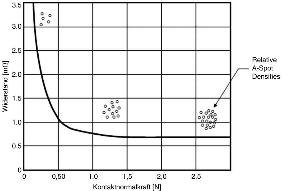
Bild 8.1 Kontaktwiderstand in Abhängigkeit von der Kontaktnormalkraft bei verzinnten Oberflächen
